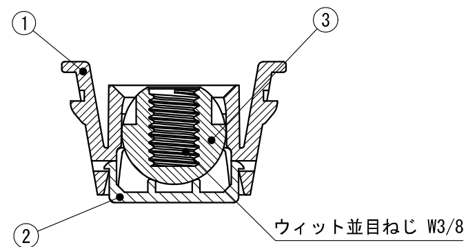
断面 A-A
